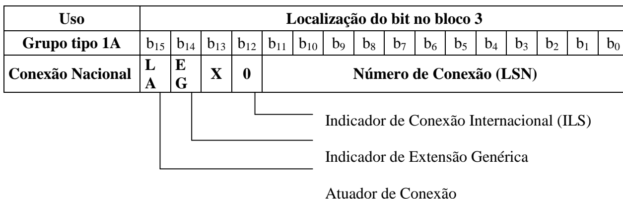
Figura 32: Estrutura Variante 12 do Bloco 3 do Grupo 14 A (informações de conexão) – Conexão Nacional
