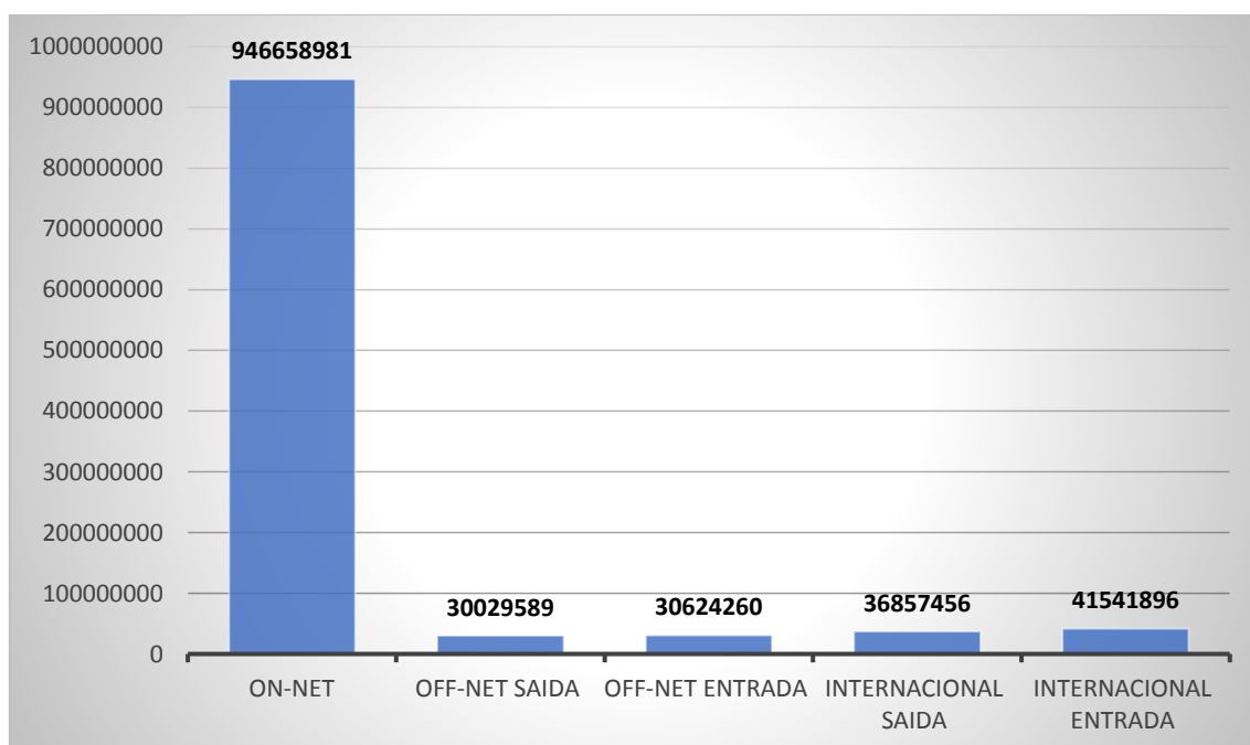
Gráfico global de repartição do tráfego de voz
