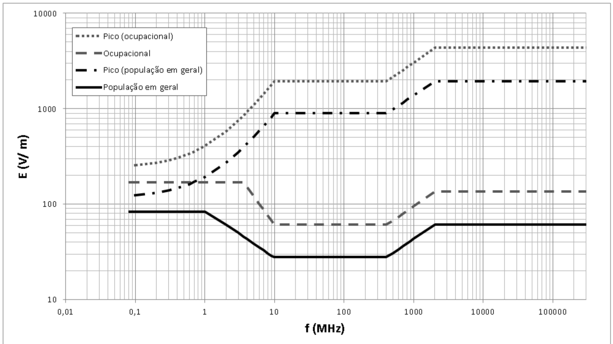
Figura A.1 – Limites para exposição humana a campos elétricos.
