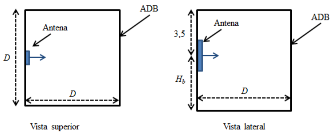
Figura B.2 – Visão da ADB para uma antena setorial. A seta na antena indica a direção de máxima radiação.
